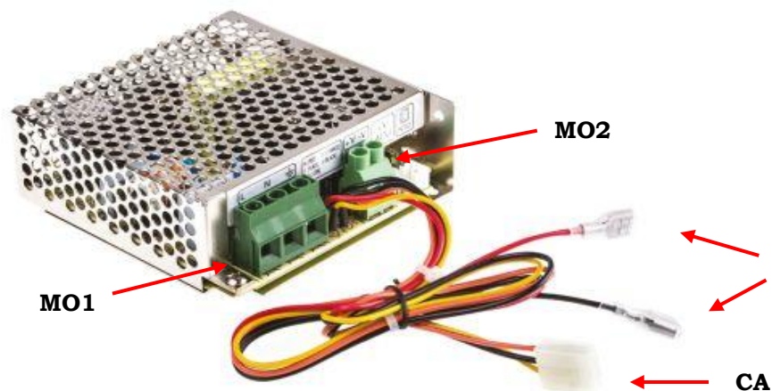
Fig. 4: alimentatore switching
